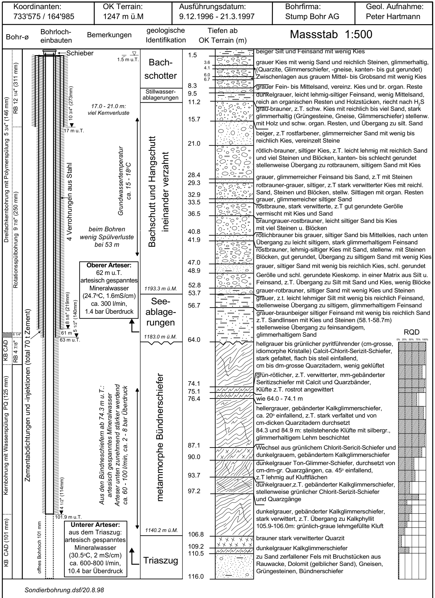
Figur 8-2: Bohrprofil der Sondierbohrung Vals
