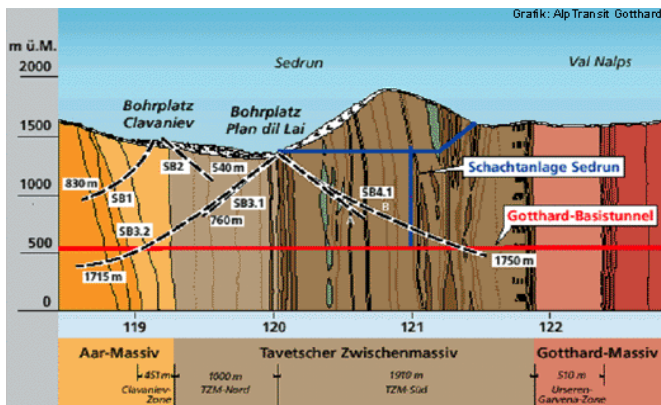
Geologischer Querschnitt durch das Sedruner Teilstück. Quelle: Arge Transco Sedrun
