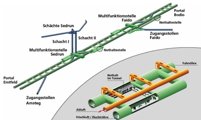
Grafische Darstellung des Tunnelsystems. Quelle: Alp Transit Gotthard AG
