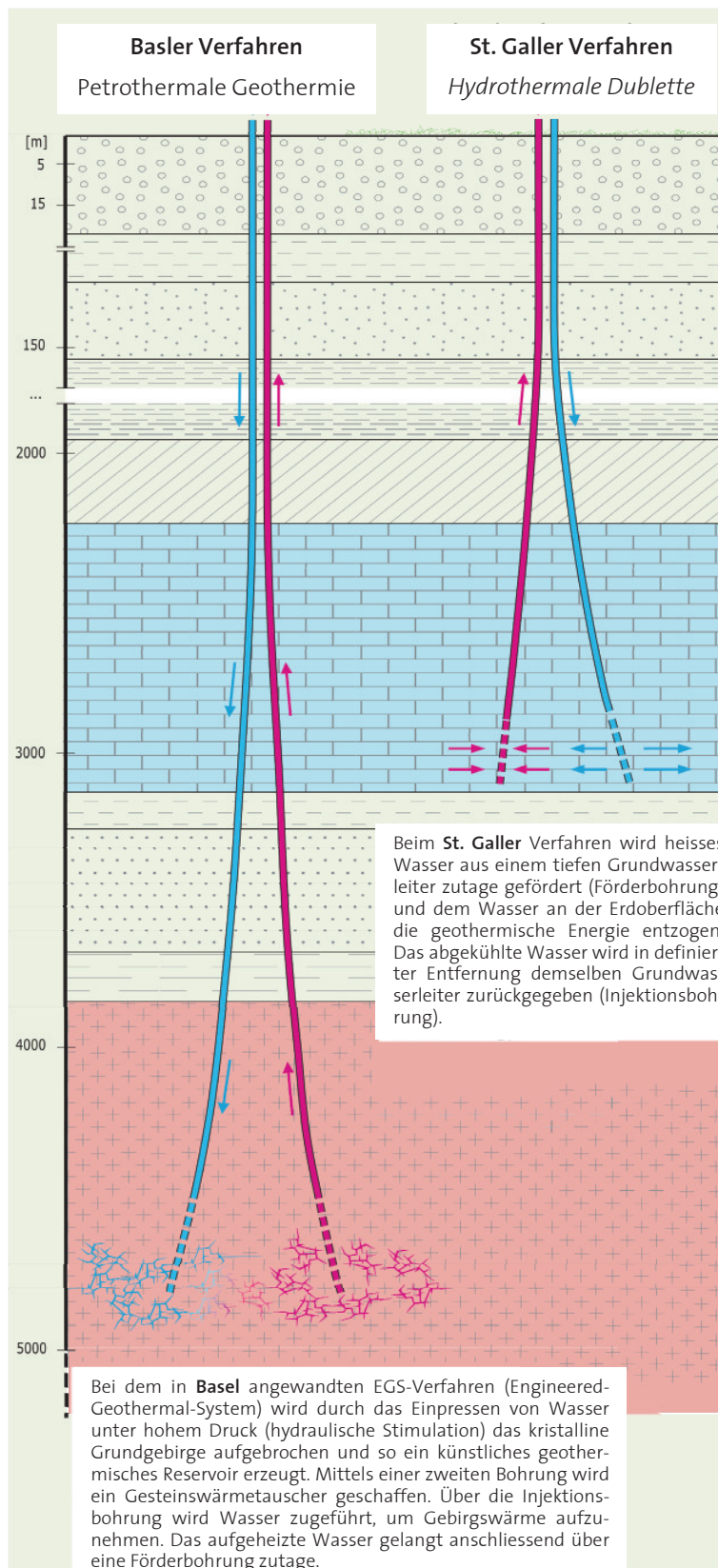
Abbildung 1: Die beiden Verfahren im graphischen Vergleich (Verändert nach: Jodocy, M., Köhler, S. & Stober, I. Geothermische Nutzungssysteme. Poster des Regierungspräsidium Freiburg, Landeshydrogeologie und -Geothermie, 2007).
